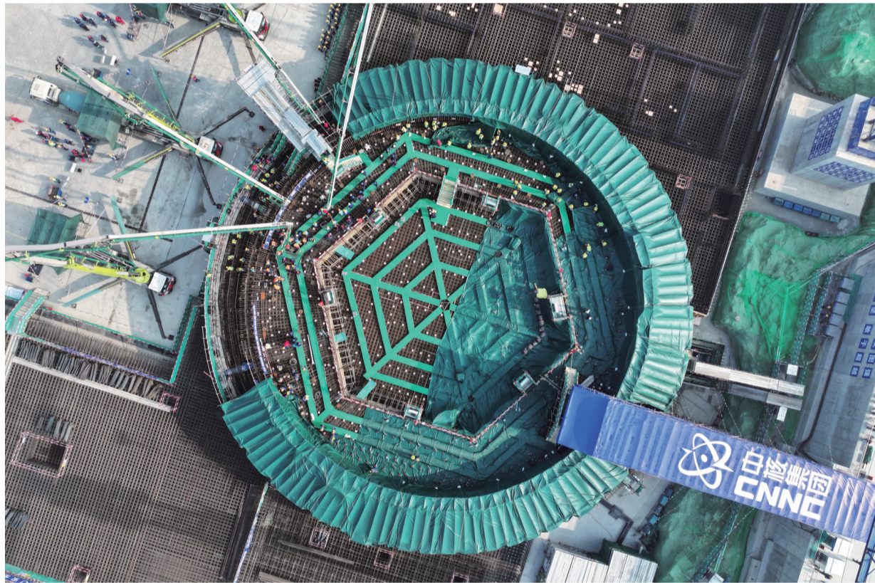
1月16日，1号机组核岛开始混凝土浇筑（无人机照片）。 1月16日，位于江苏省连云港市的江苏徐圩核能供热发电厂1号机组核岛开始混凝土浇筑，项目进入主体工程建设阶段。这是“十五五”开局之年我国开工建设的首台核电机组。 新华社记者 毛俊 摄
